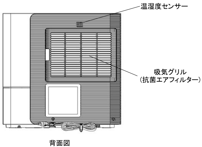
背面図
