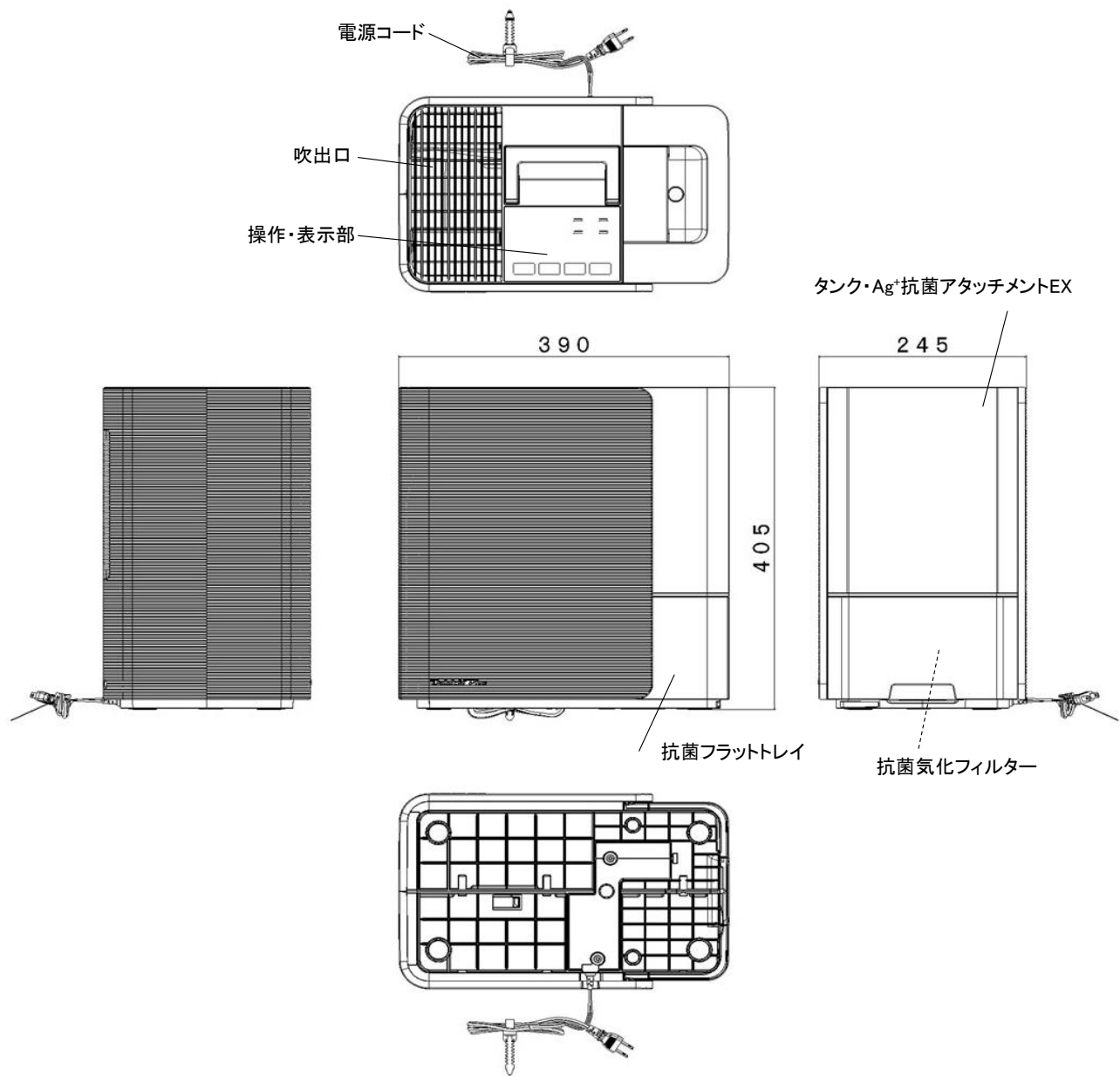
外形寸法図
