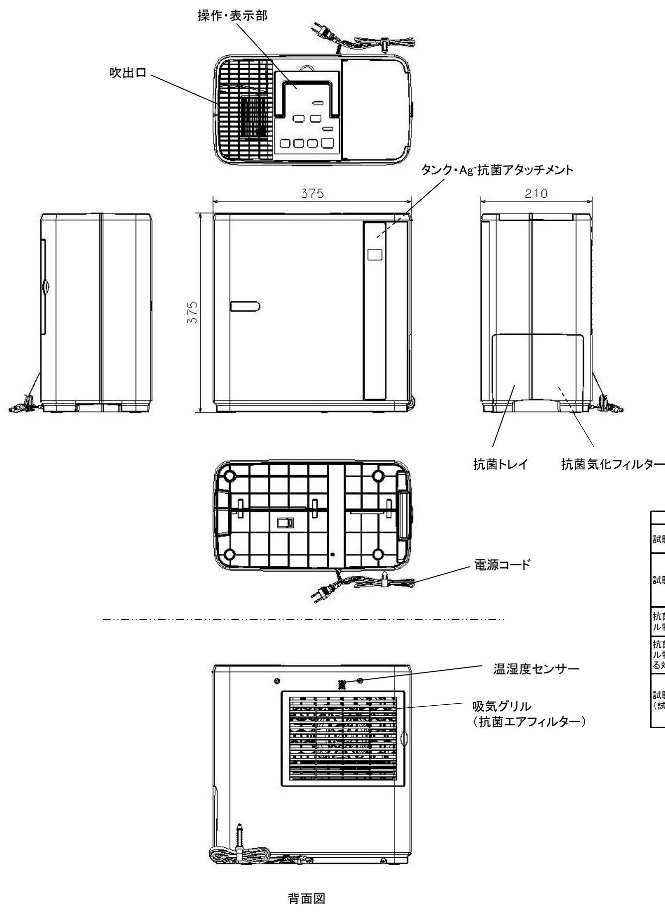
外形寸法図
