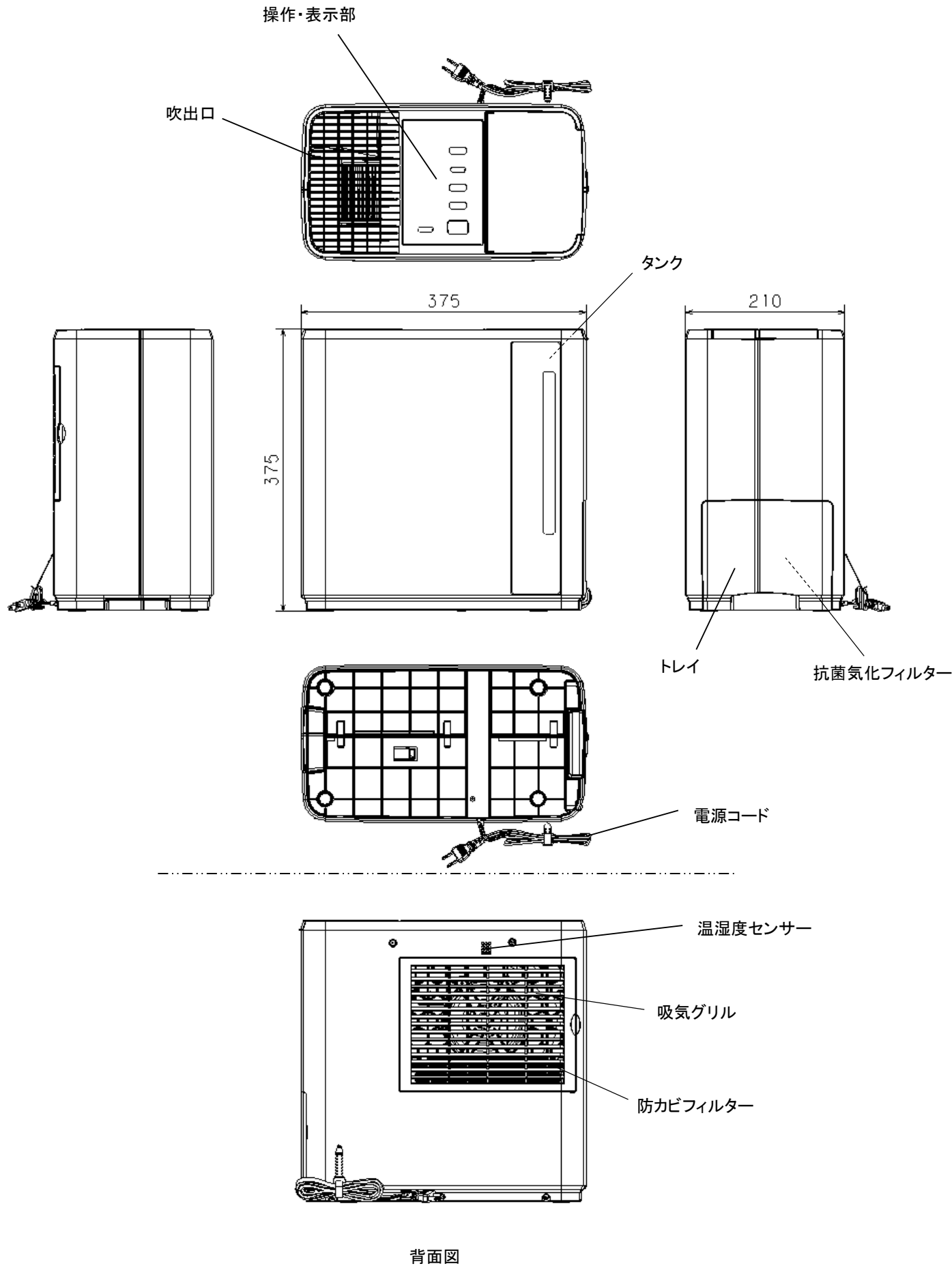
外形寸法図
