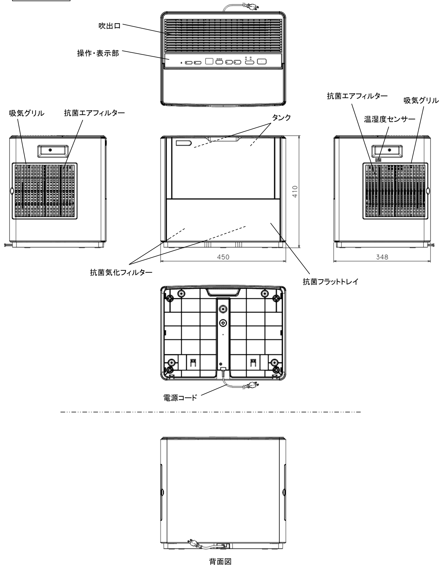
外形寸法図
