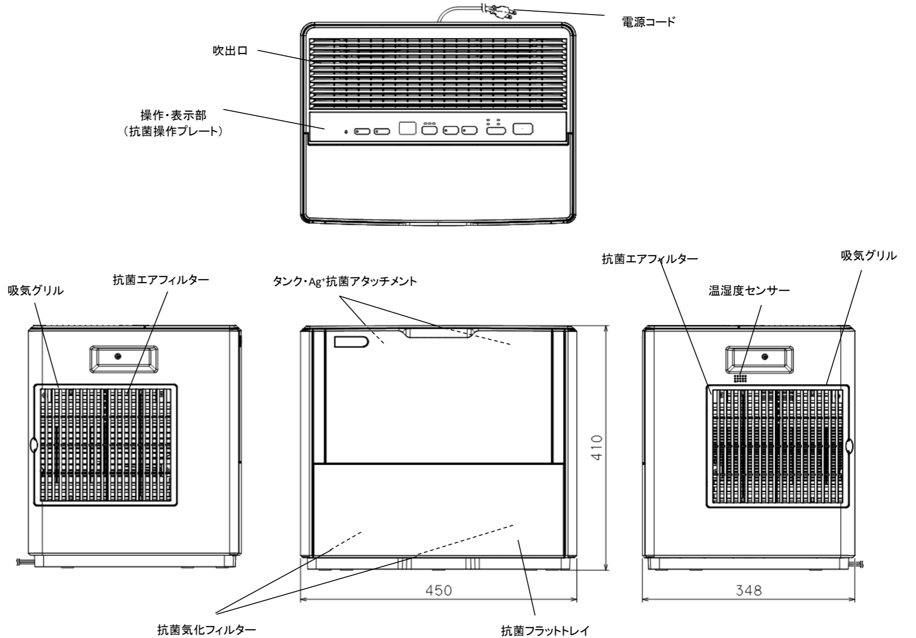
外形寸法図
