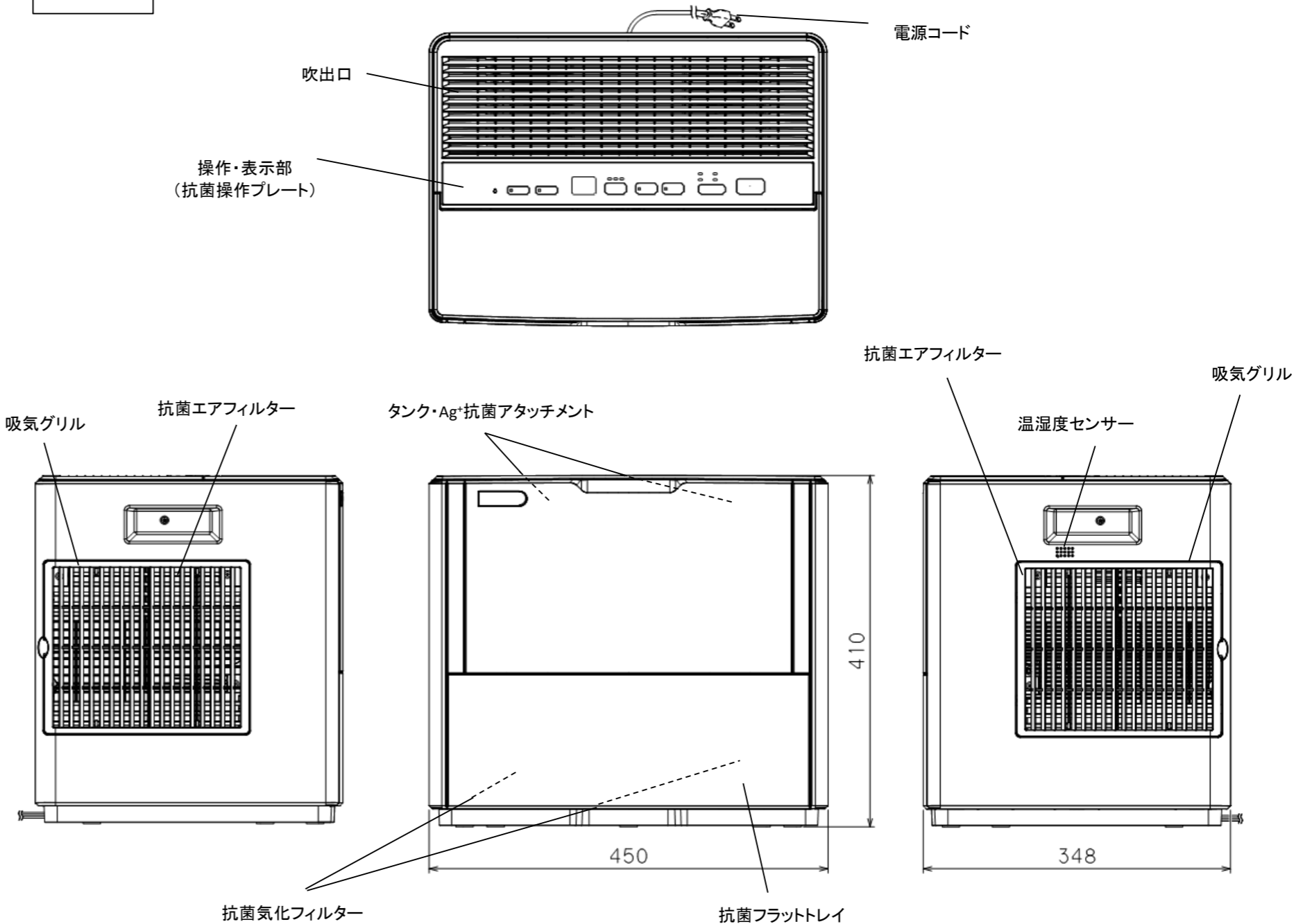
外形寸法図
