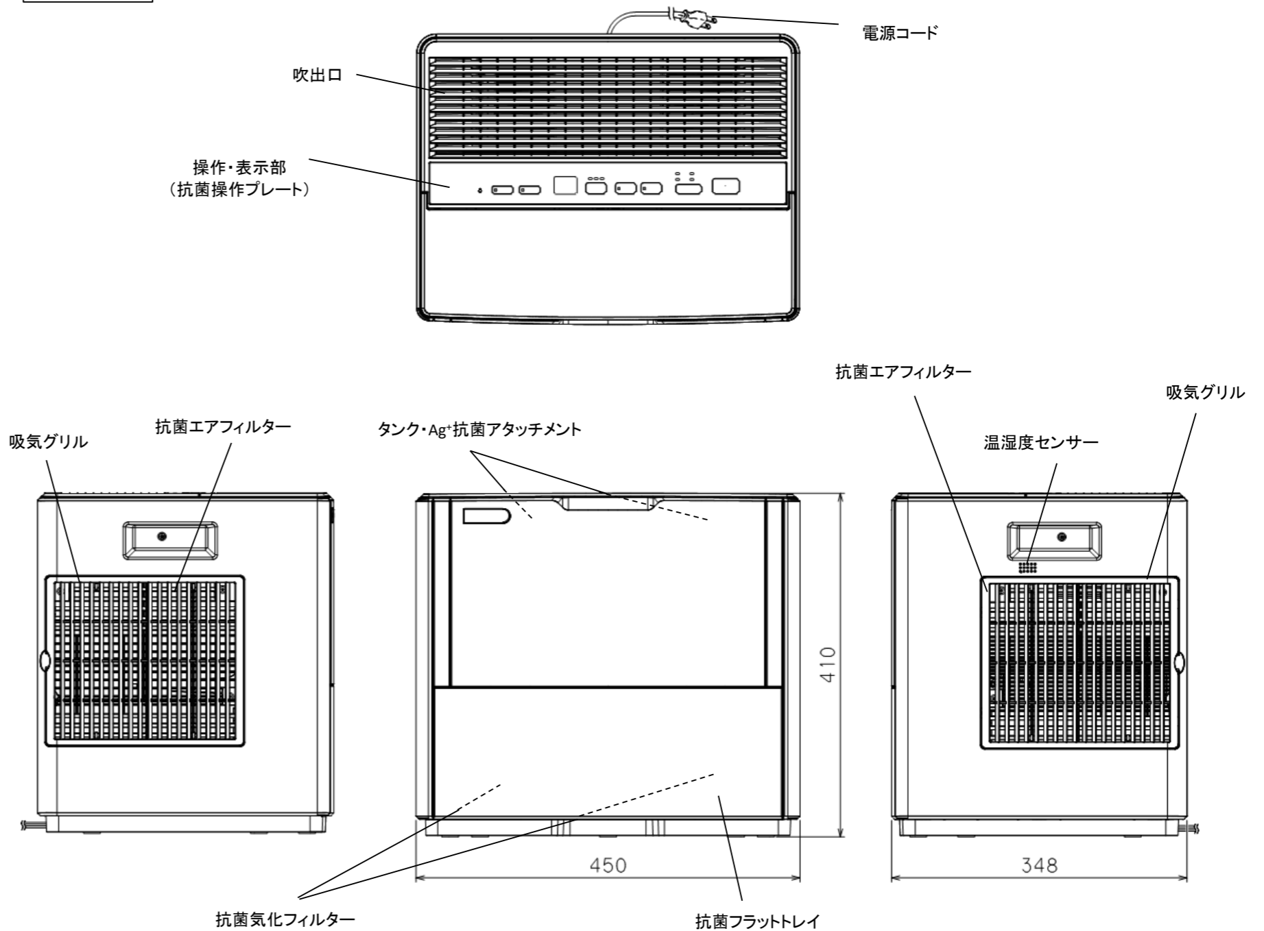
外形寸法図
