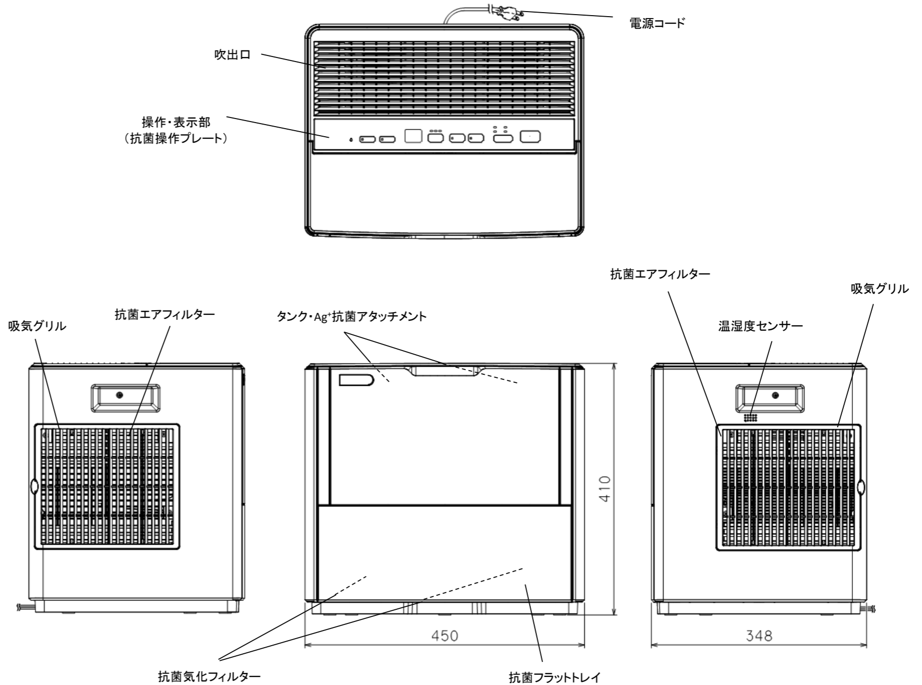
外形寸法図
