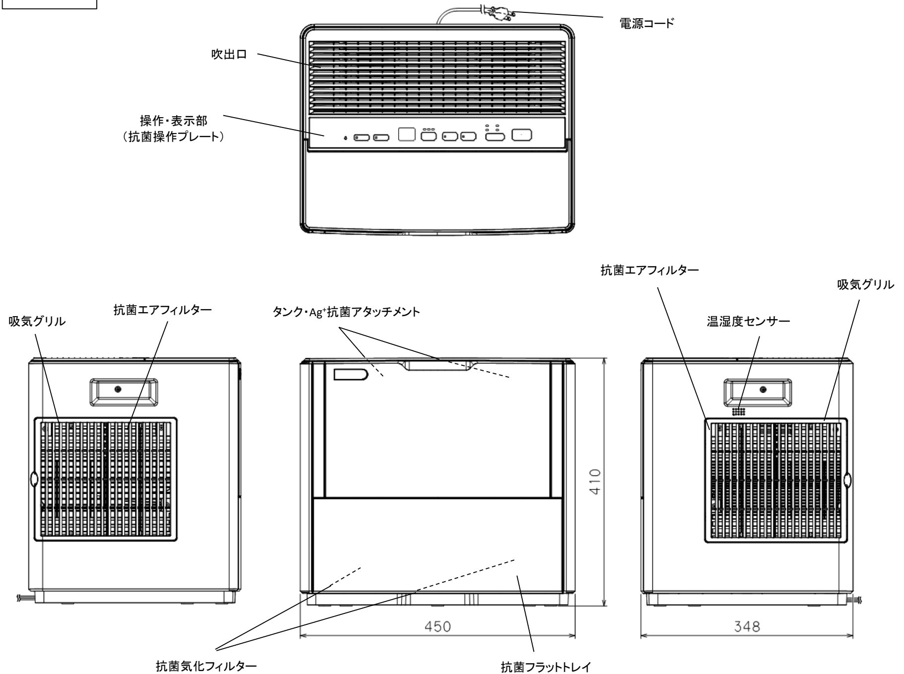
外形寸法図
