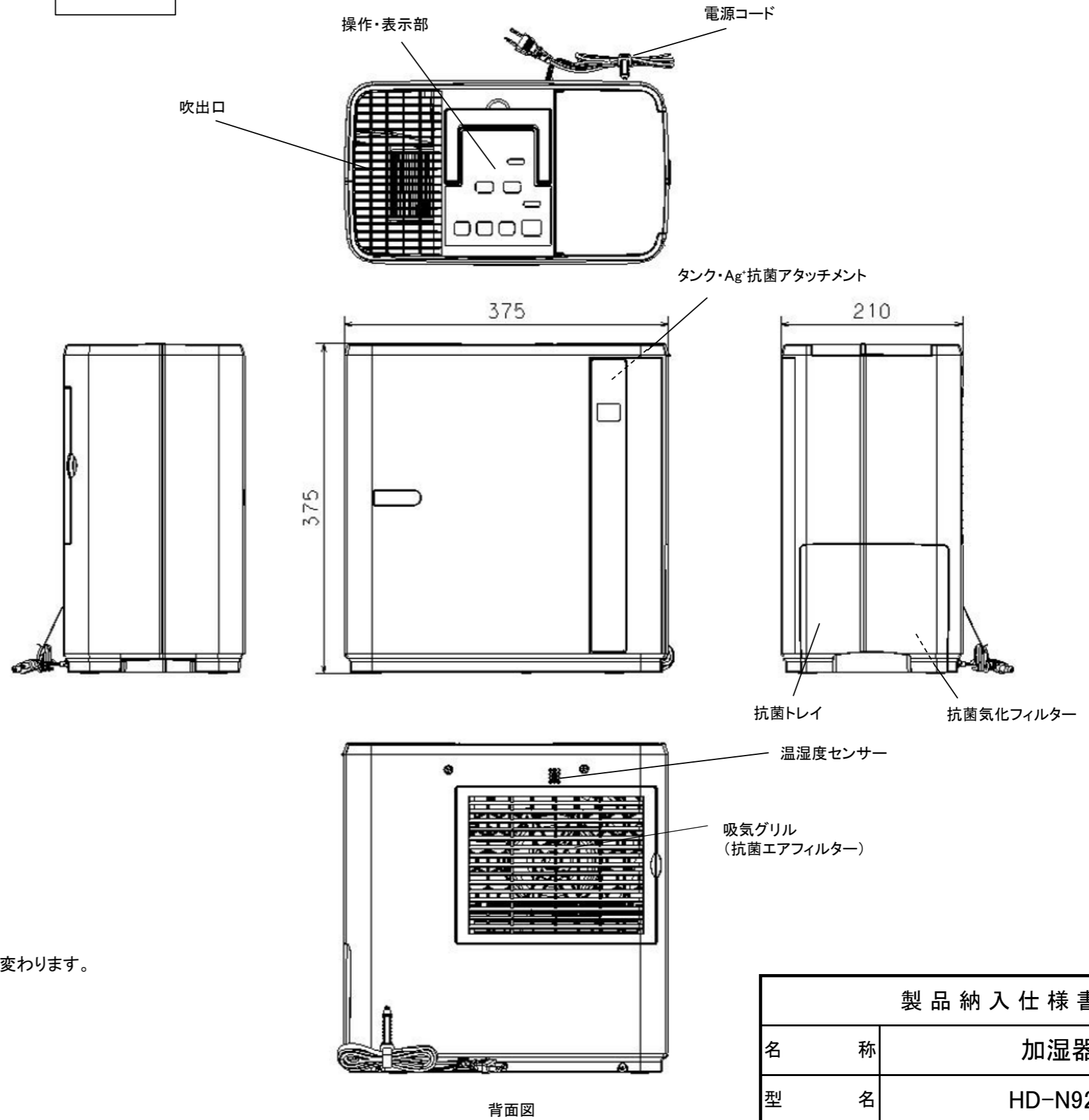
外形寸法図
