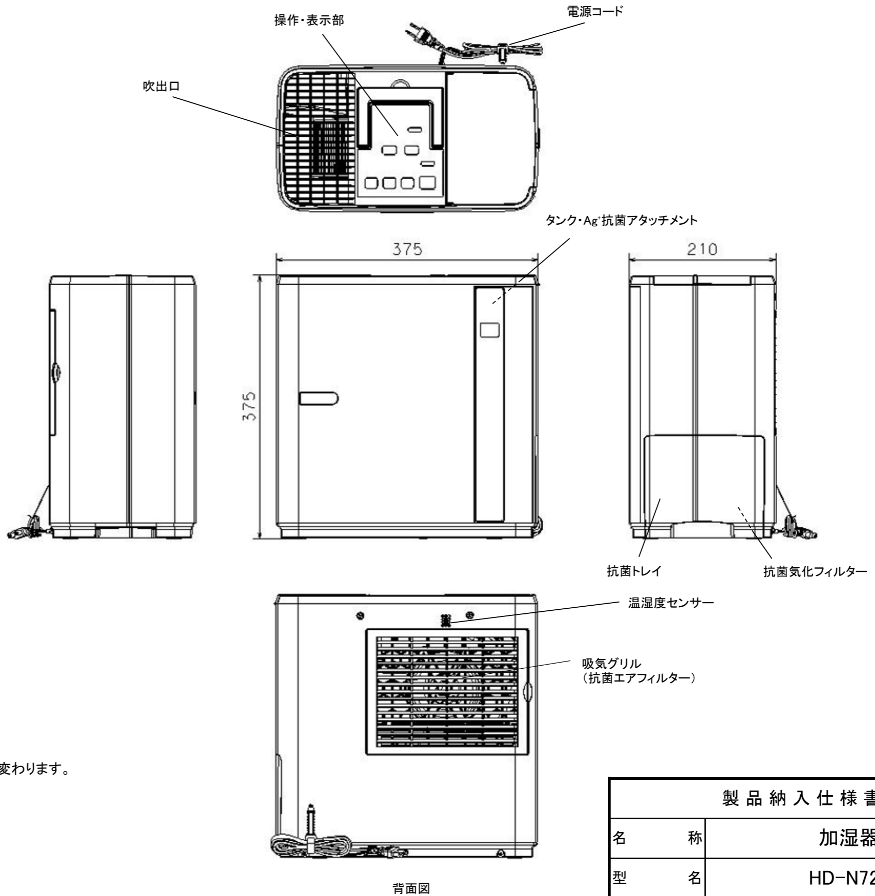
外形寸法図
