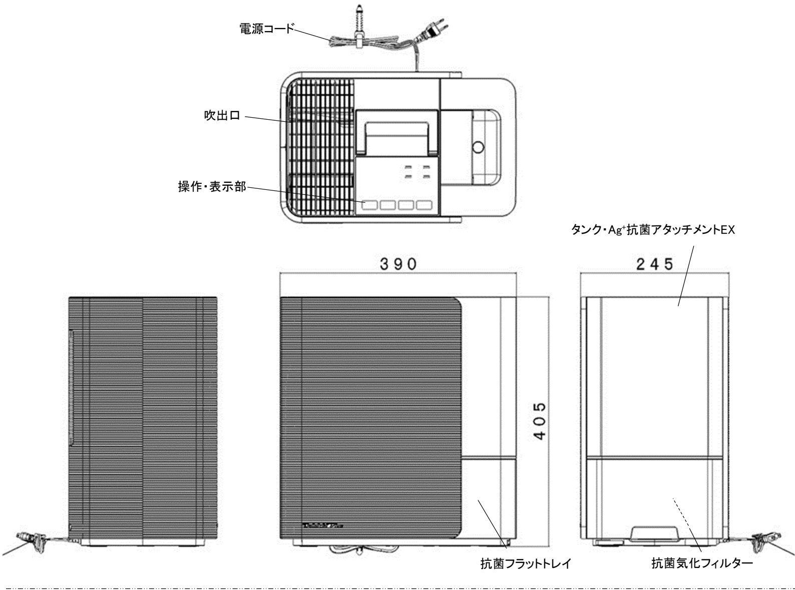
外形寸法図
