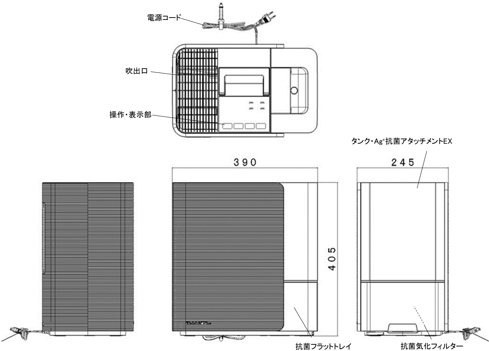
外形寸法図
