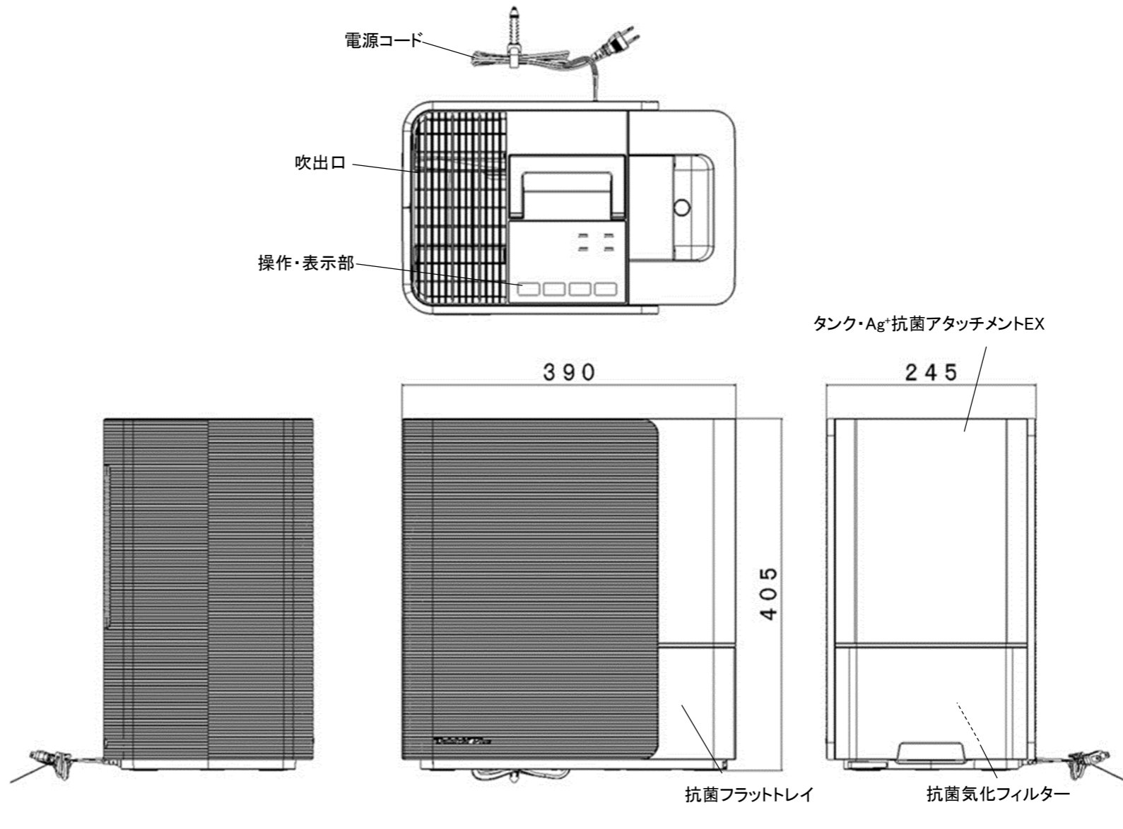
外形寸法図
