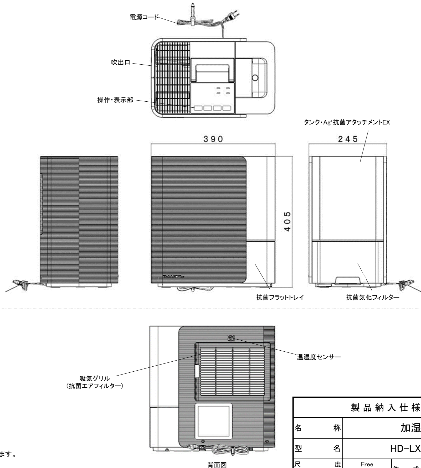
外形寸法図
