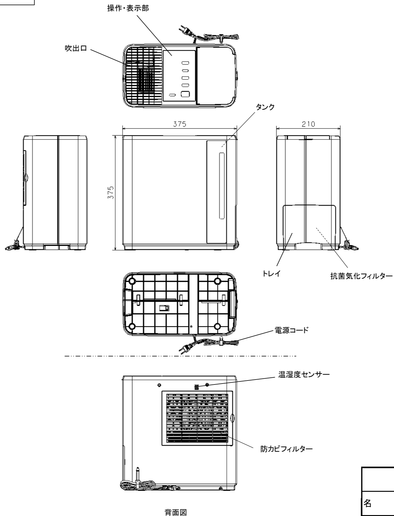
外形寸法図
