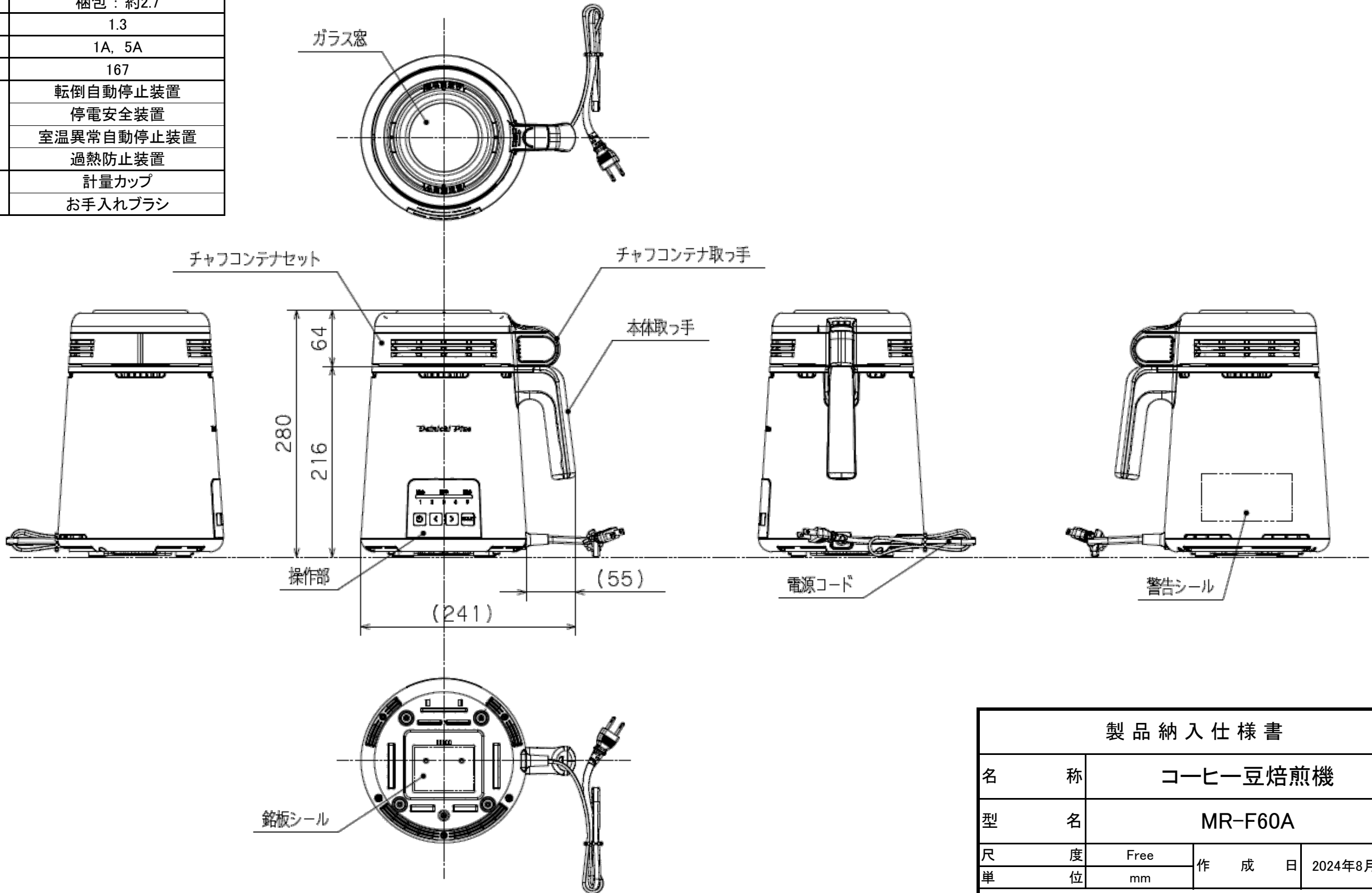
外形寸法図
