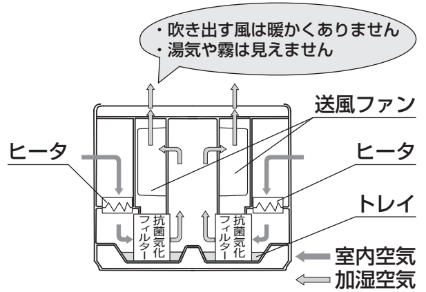
※イラストはHD-PC2400Gで説明しています。左側のヒータはHD-PC2400Gのみです。
