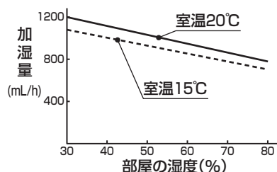
部屋の湿度と加湿量 (標準運転のとき)
