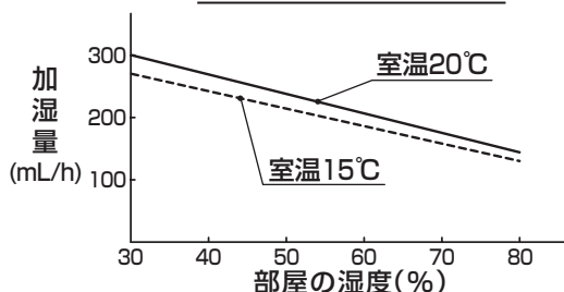
部屋の湿度と加湿量 (標準運転モードのとき)
