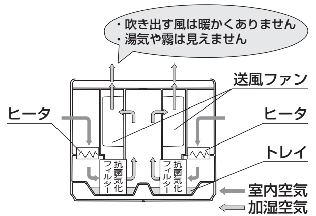
※イラストはHD-PN246で説明しています。 左側のヒータはHD-PN246のみです。
