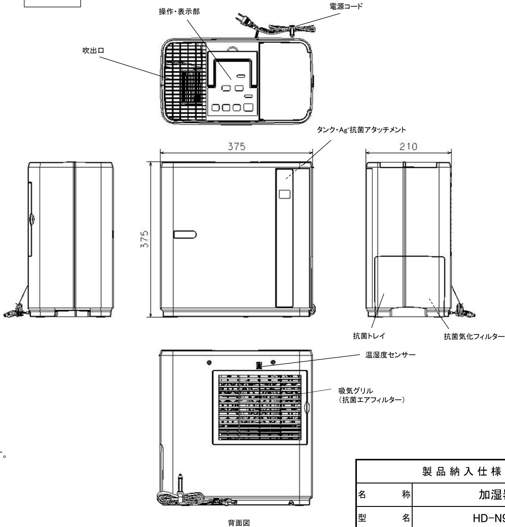
外形寸法図
