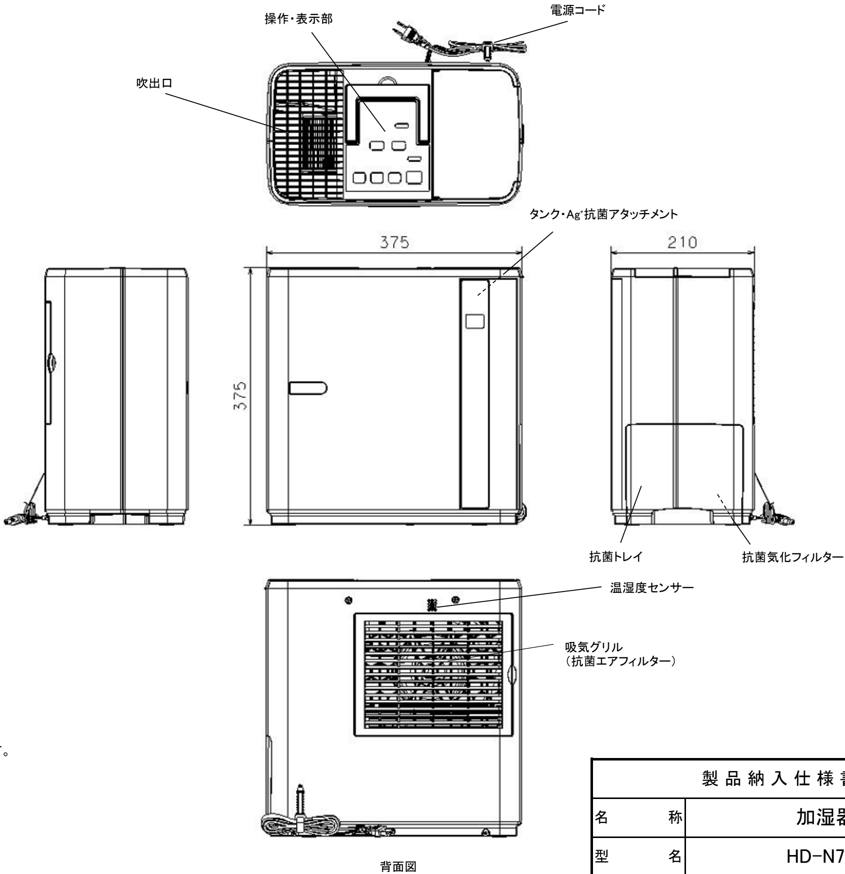
外形寸法図
