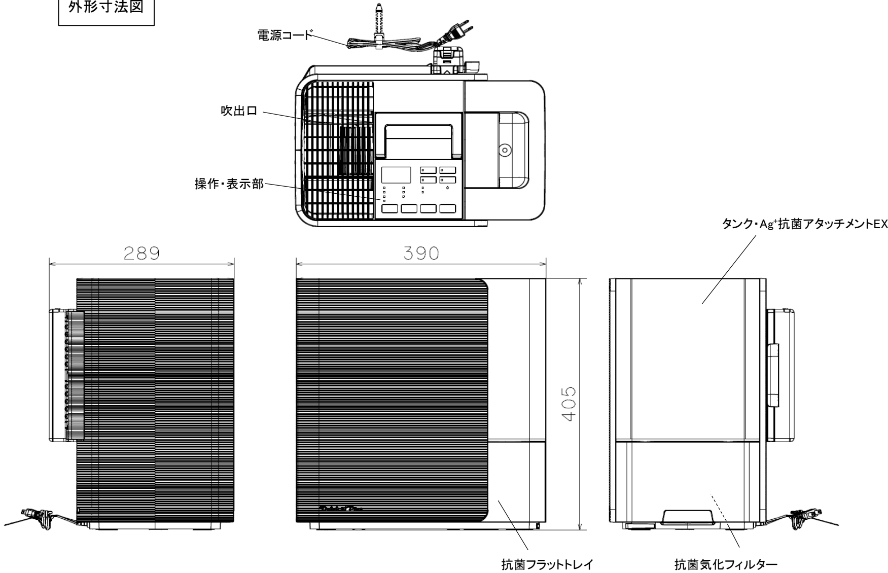
外形寸法図
