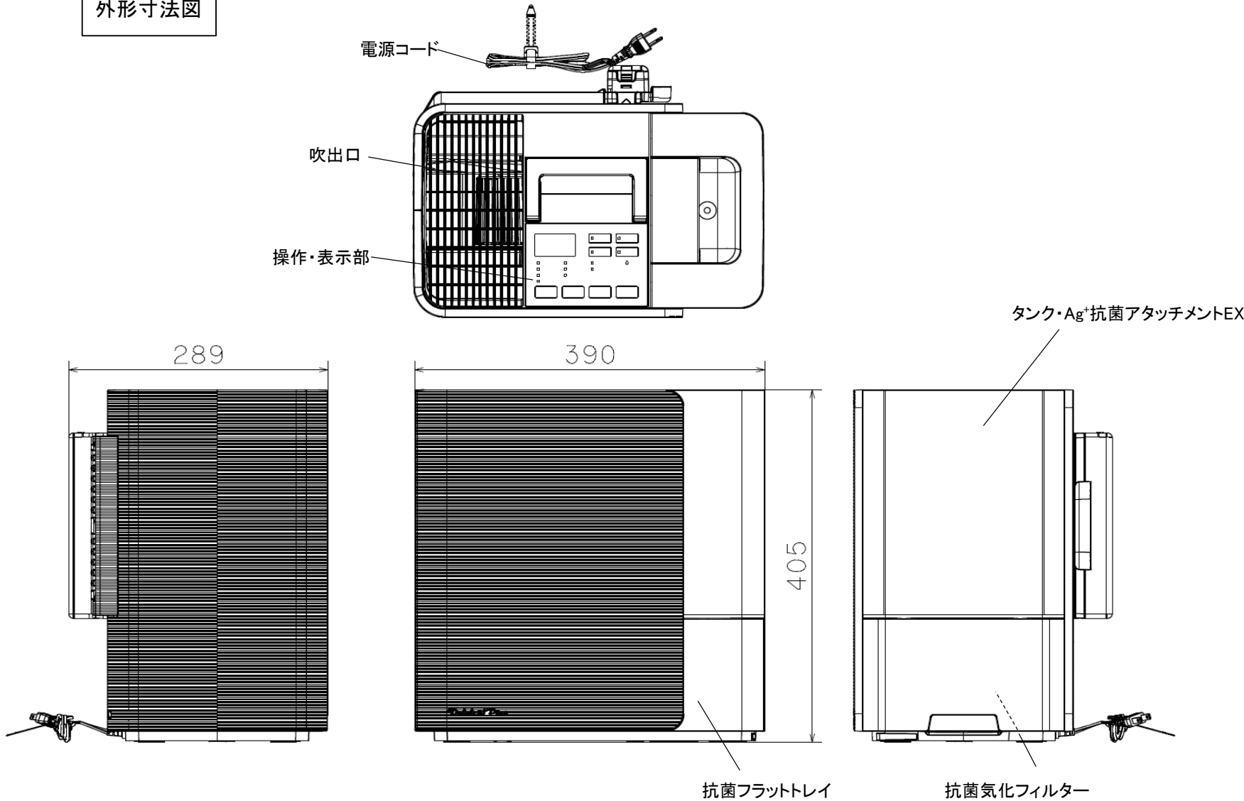
外形寸法図
