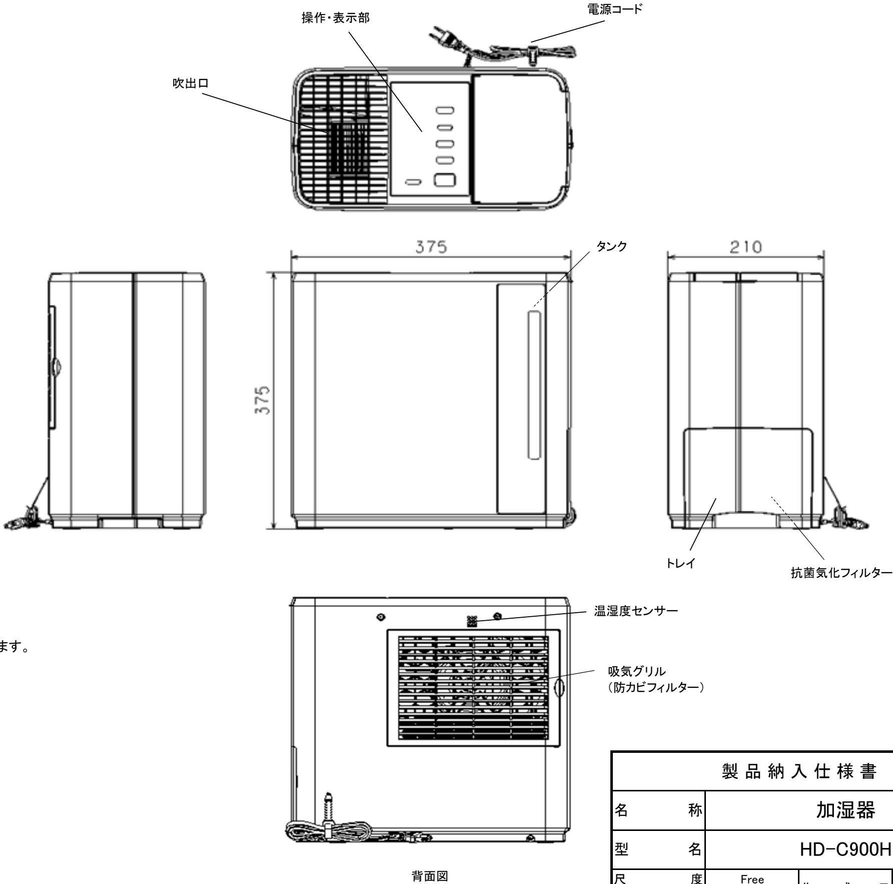
外形寸法図
