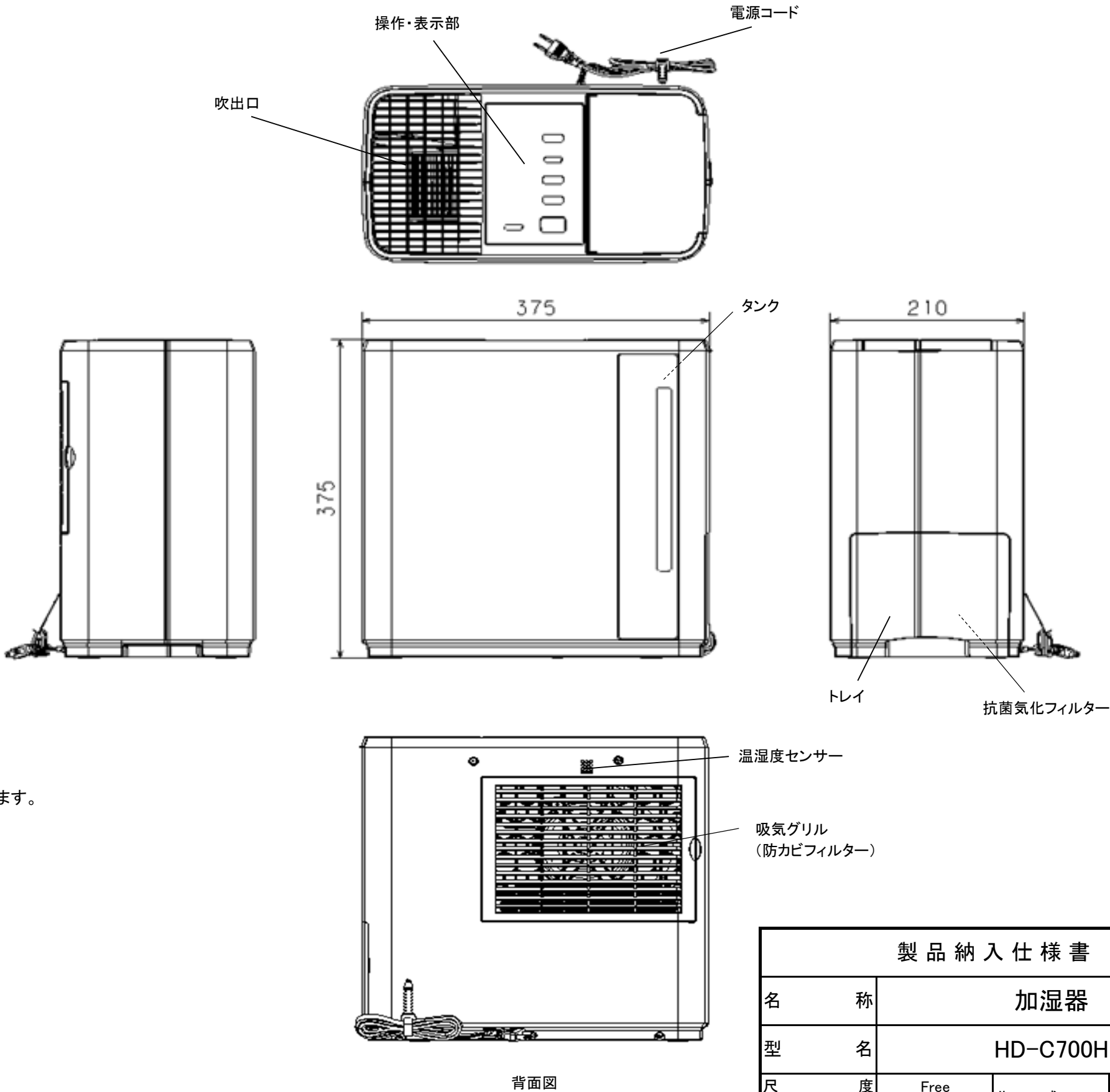
外形寸法図
