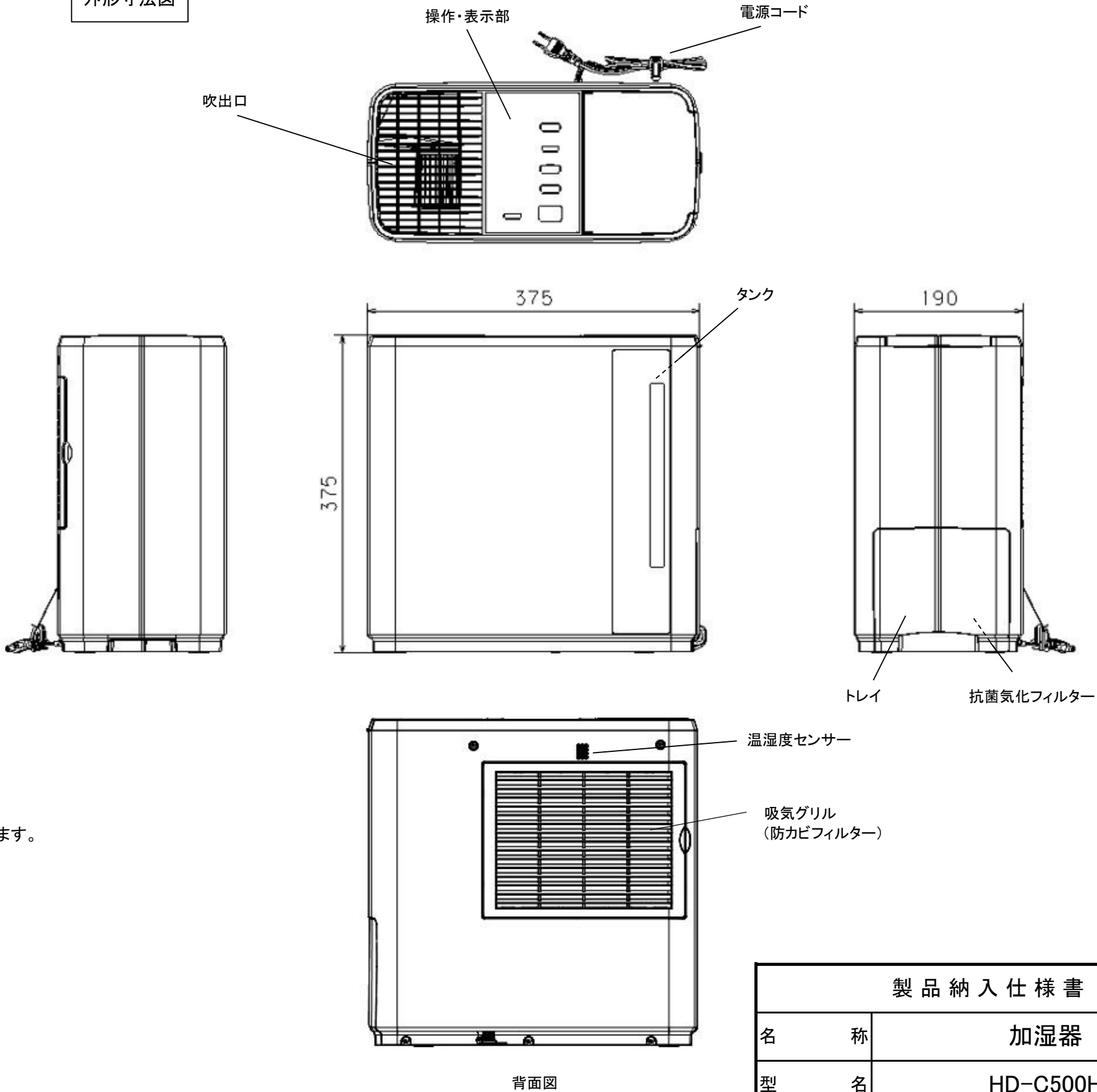
外形寸法図
