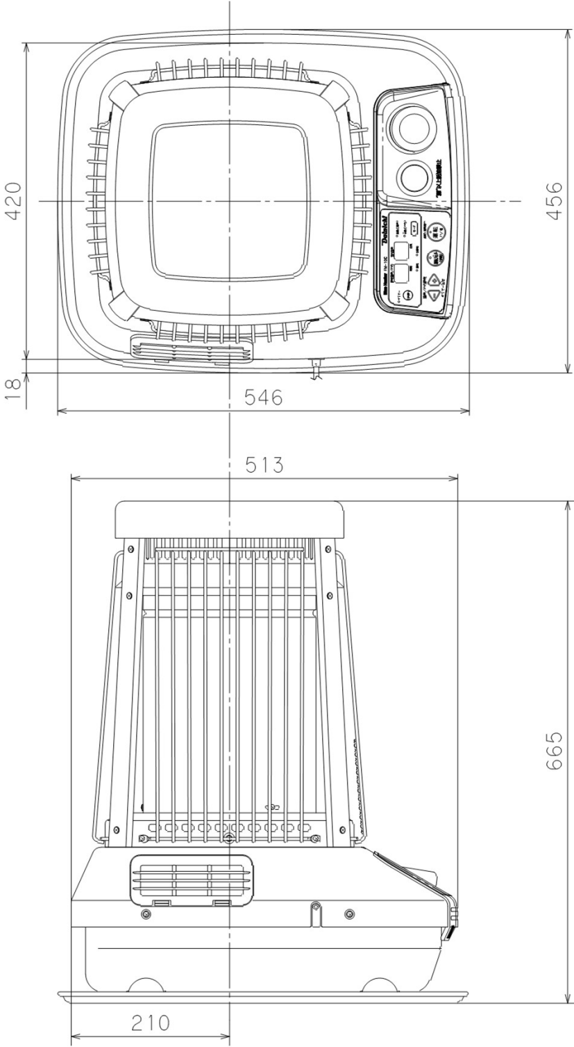
外形寸法図
