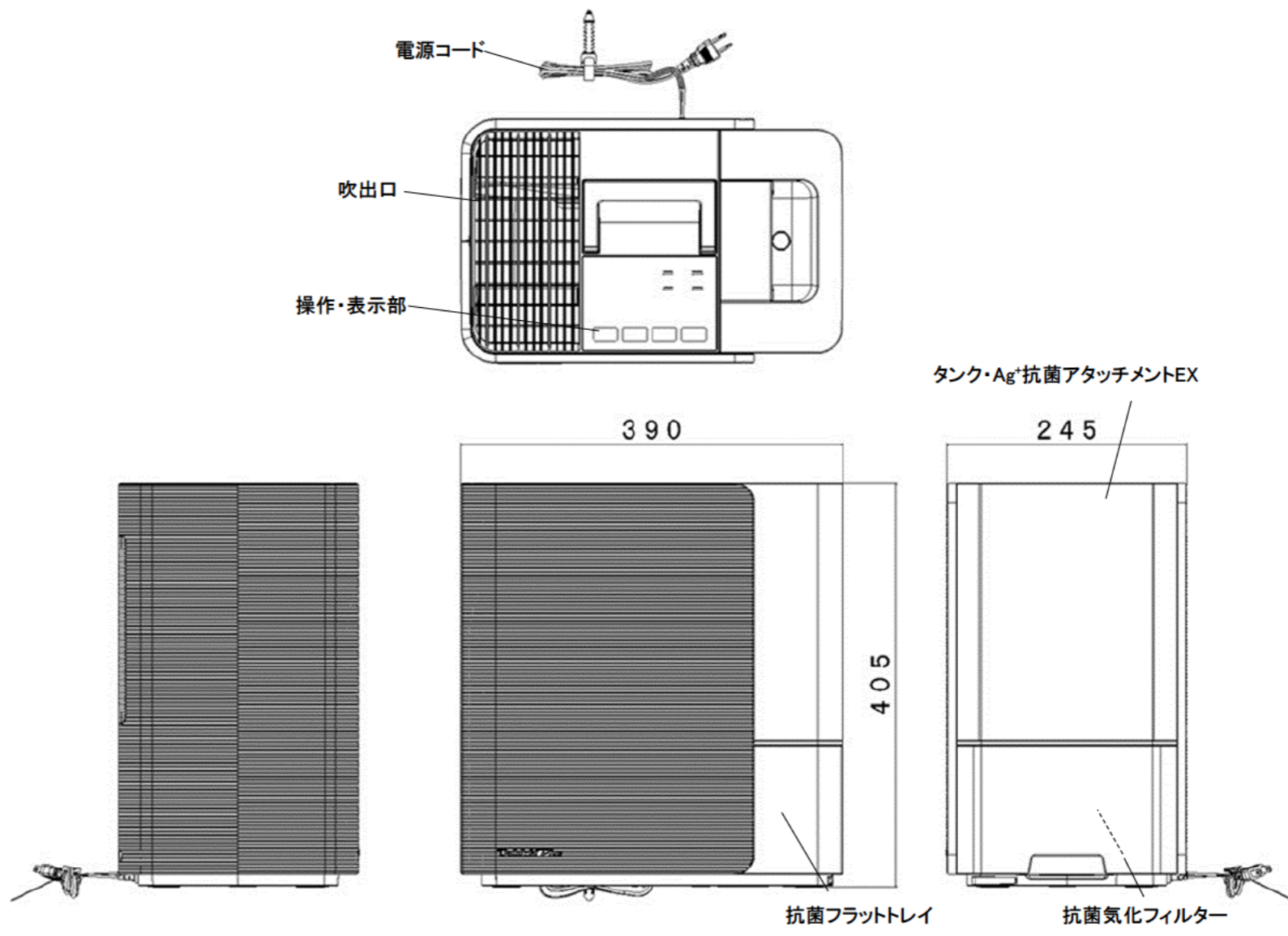
外形寸法図
