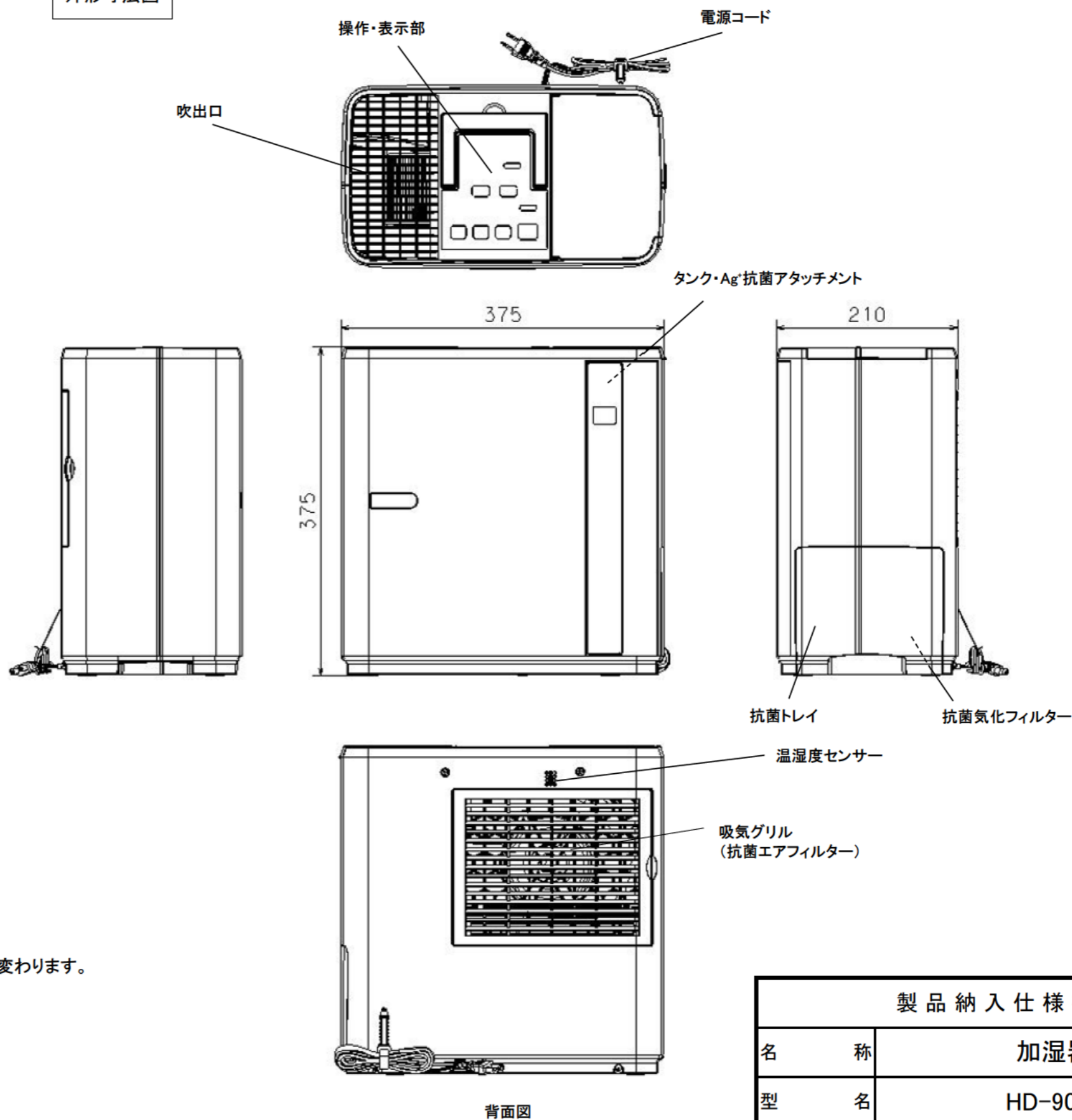
外形寸法図
