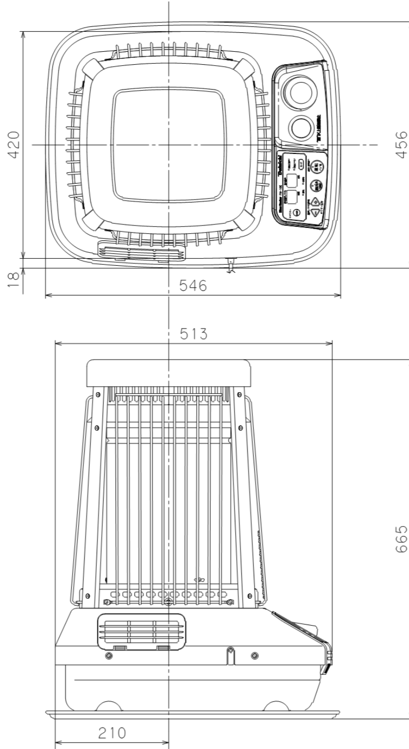
外形寸法図
