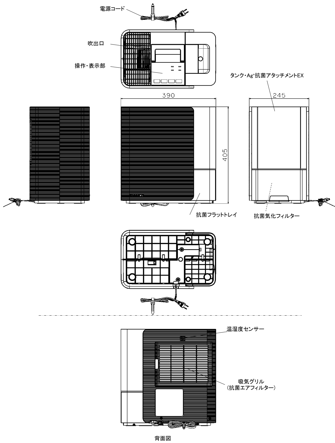
外形寸法図
