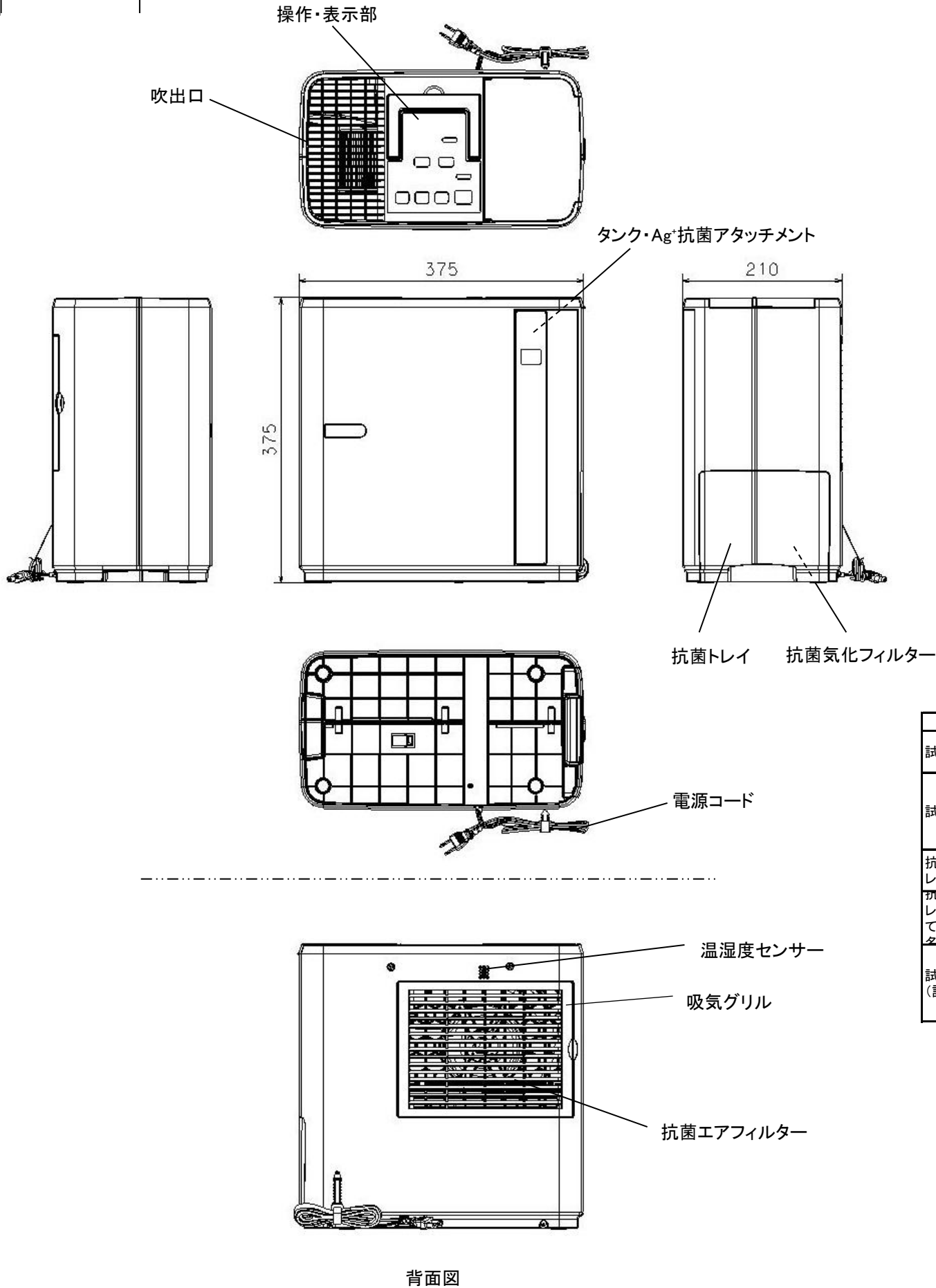
外形寸法図
