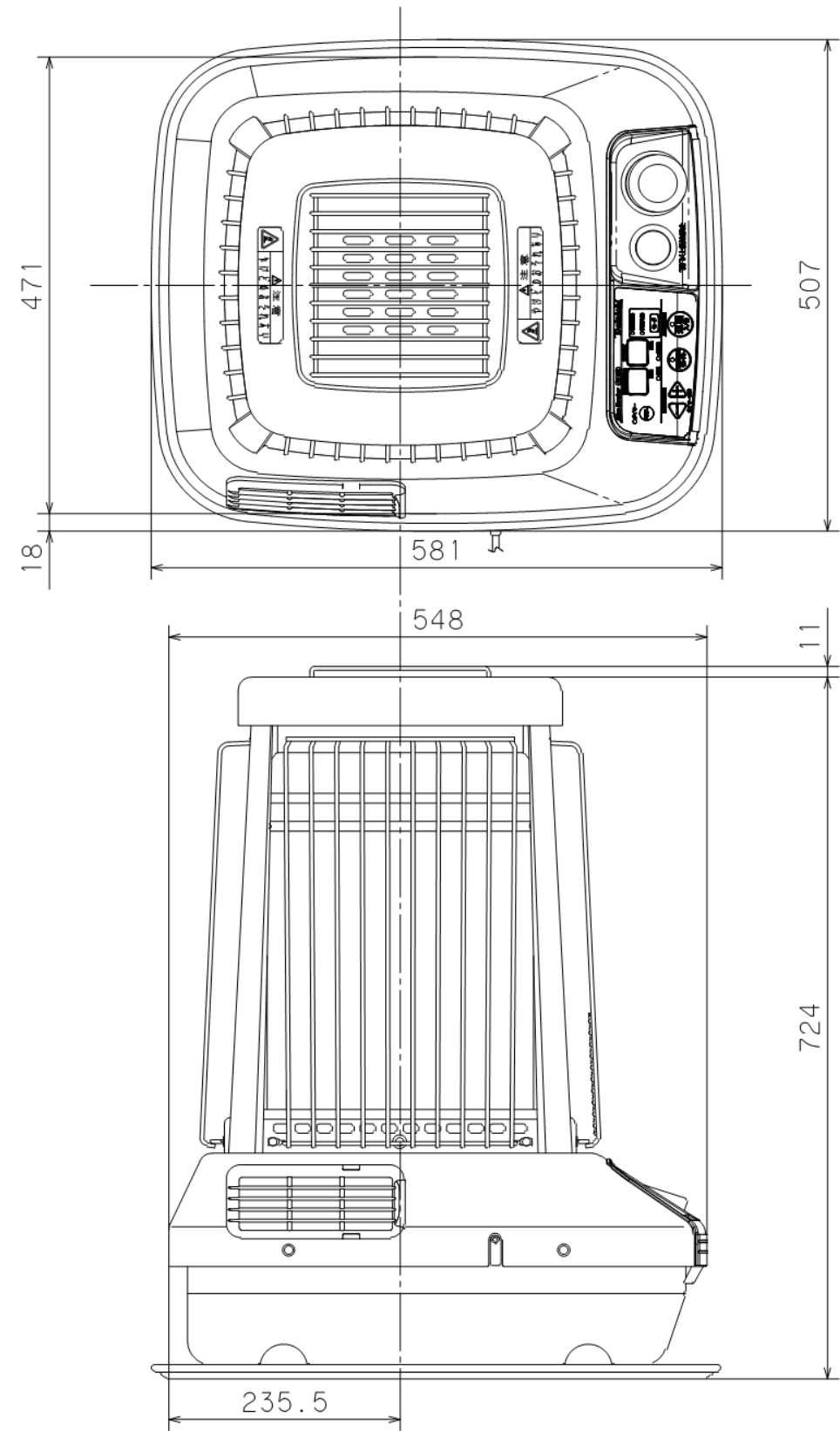
外形寸法図
