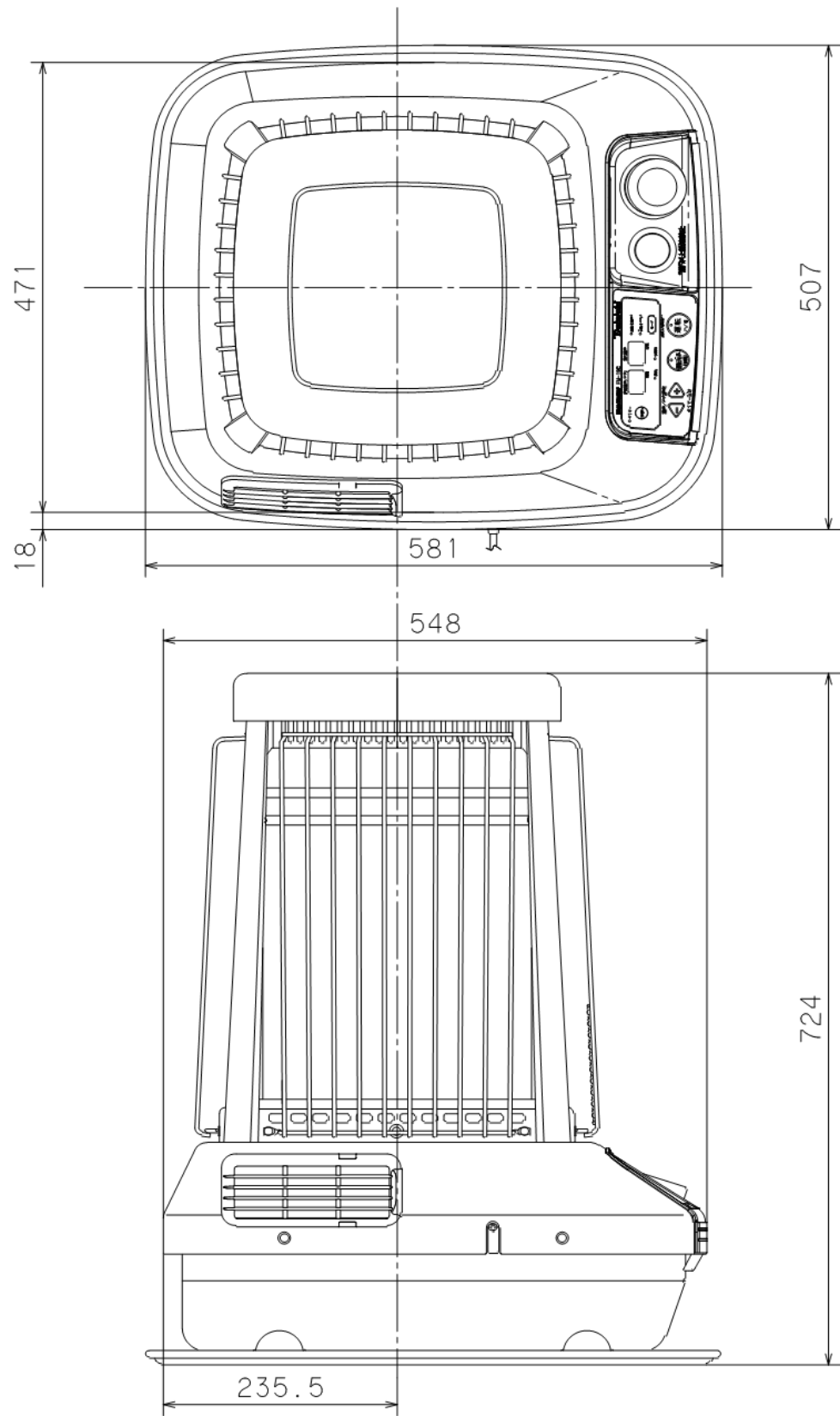
外形寸法図
