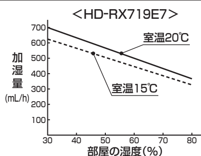
部屋の湿度と加湿量(標準運転のとき)
