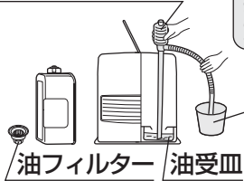
市販の給油ポンプ
