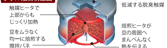
ダブル焙煎構造図
