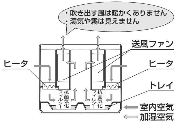
※イラストはHD-242で説明しています。 左側のヒータはHD-242のみです。
